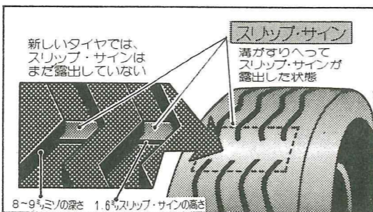
8-9ミリの深さ 1.6スリップ・サインの高さ
