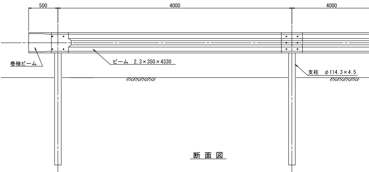
側面図
