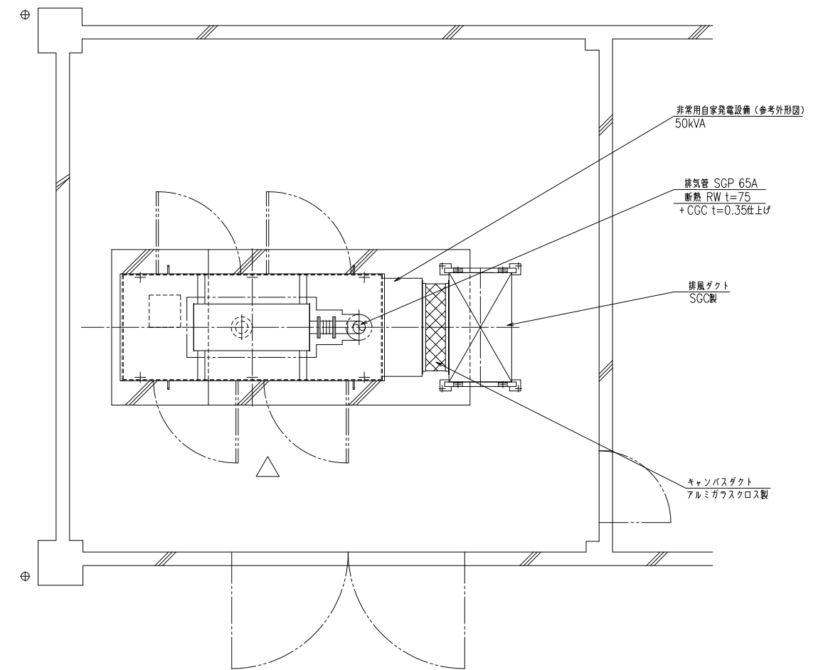
発電機室 機器配置平面図 (下部) S=None
