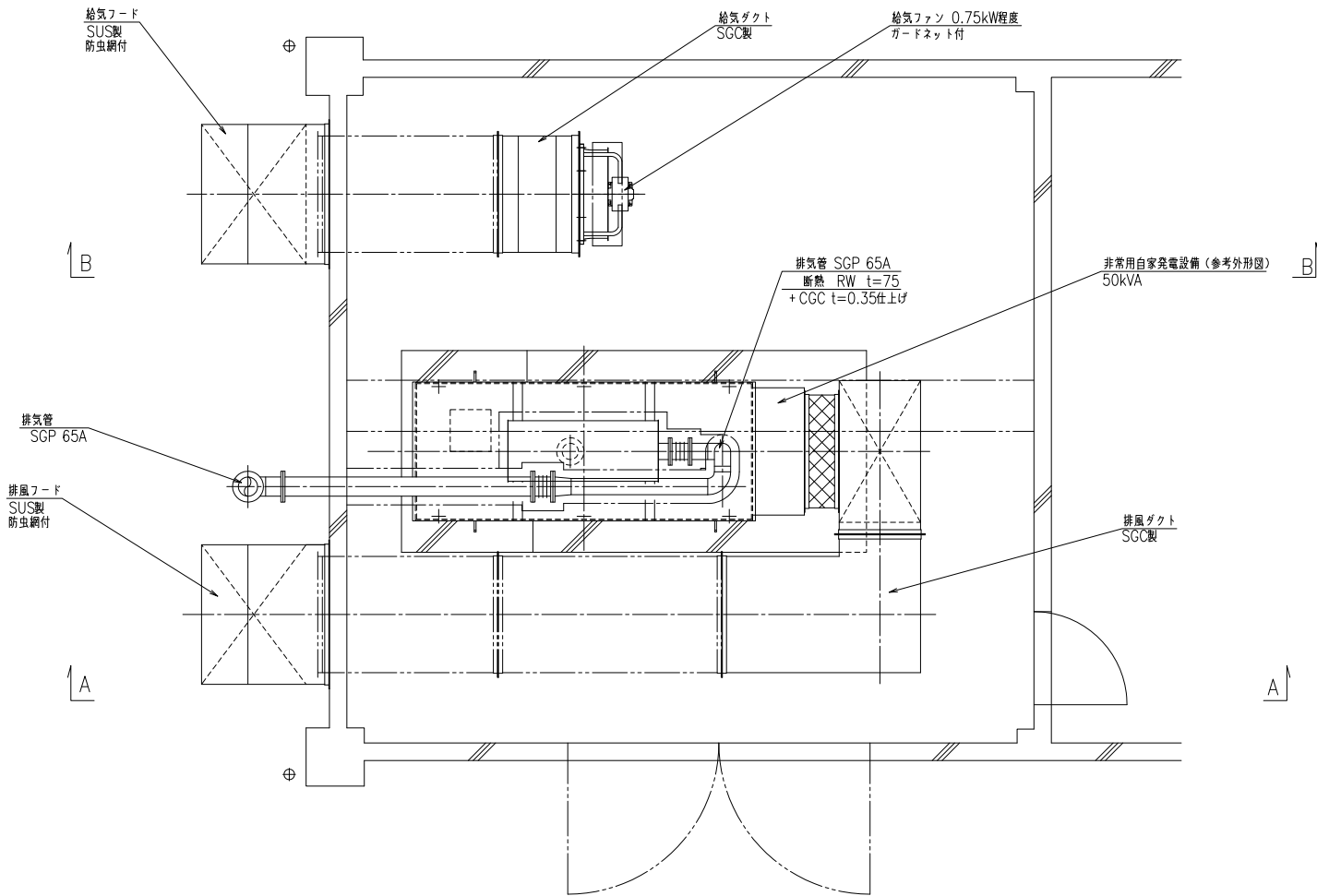
発電機室 機器配置平面図 (上部) S=None
