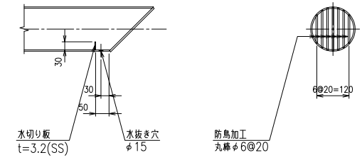
排気管 先端部詳細図 S=None
