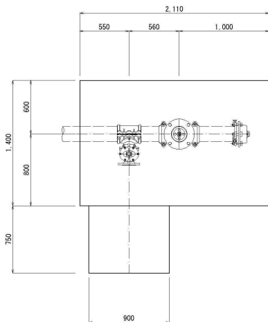
φ150×100, φ150 (既設鑄鉄管)
