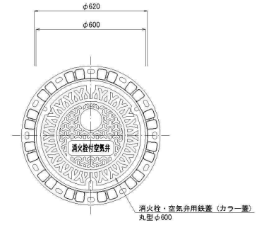
空気弁室 DP=800
