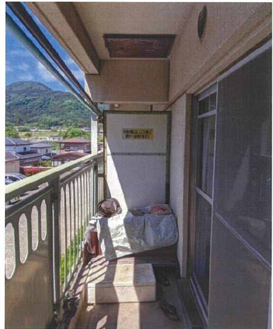
避難ハッチ操作空間確保のために室外機移設
