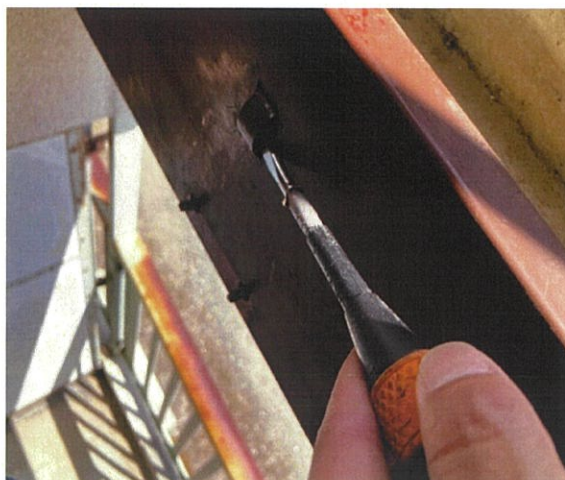
避難ハッチを閉めるピンの故障
