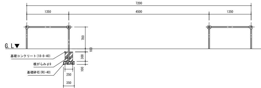
C部詳細図
