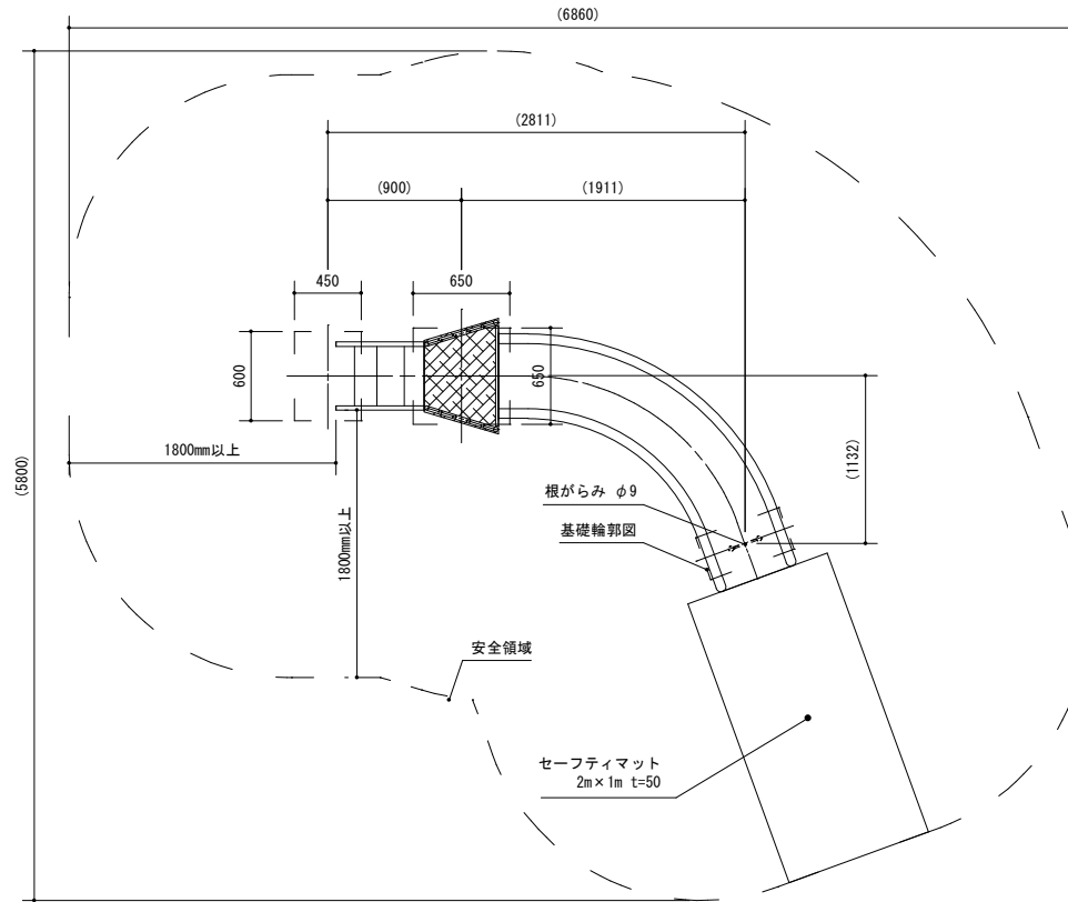
すべり台(カーブ)詳細図
