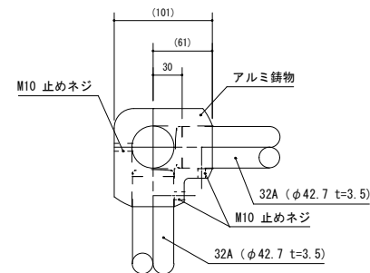
C部詳細図
