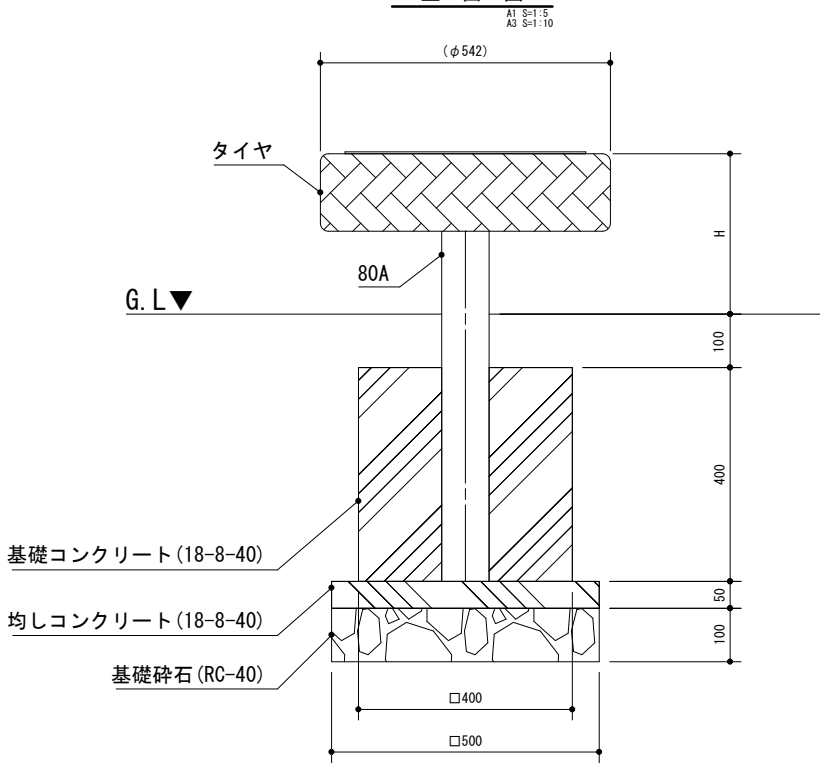
立面図
