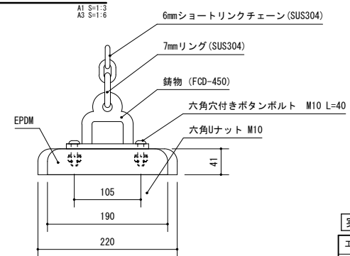
C部詳細図
