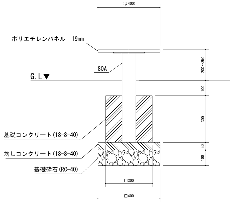
立面図
