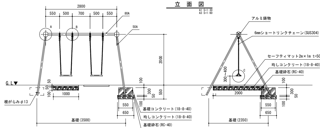
立面図
