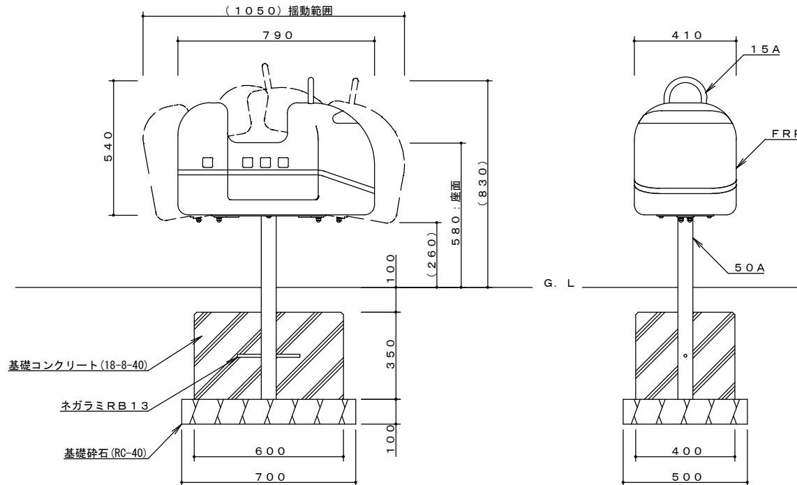
立面图
