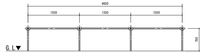
B部断面図
