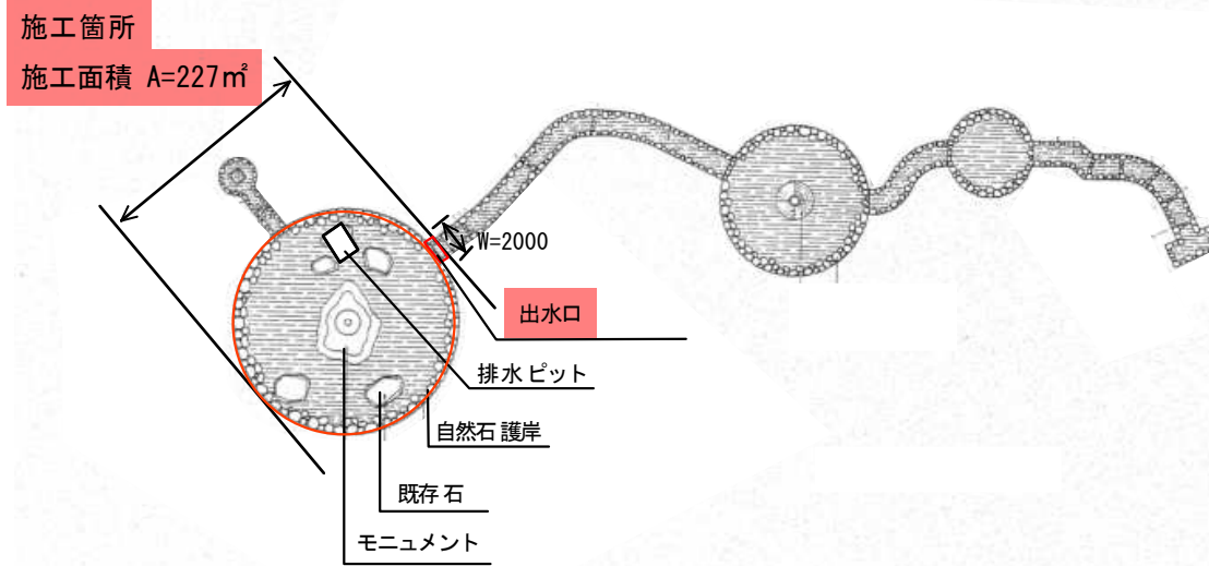
平面図
