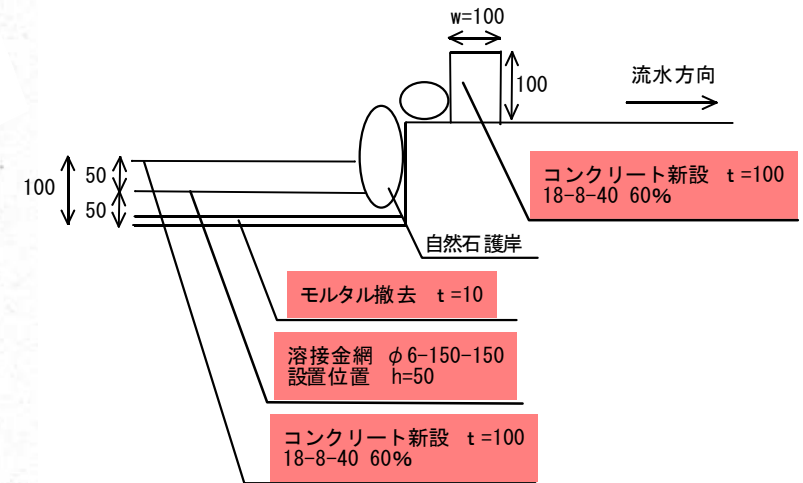
出水部断面図
